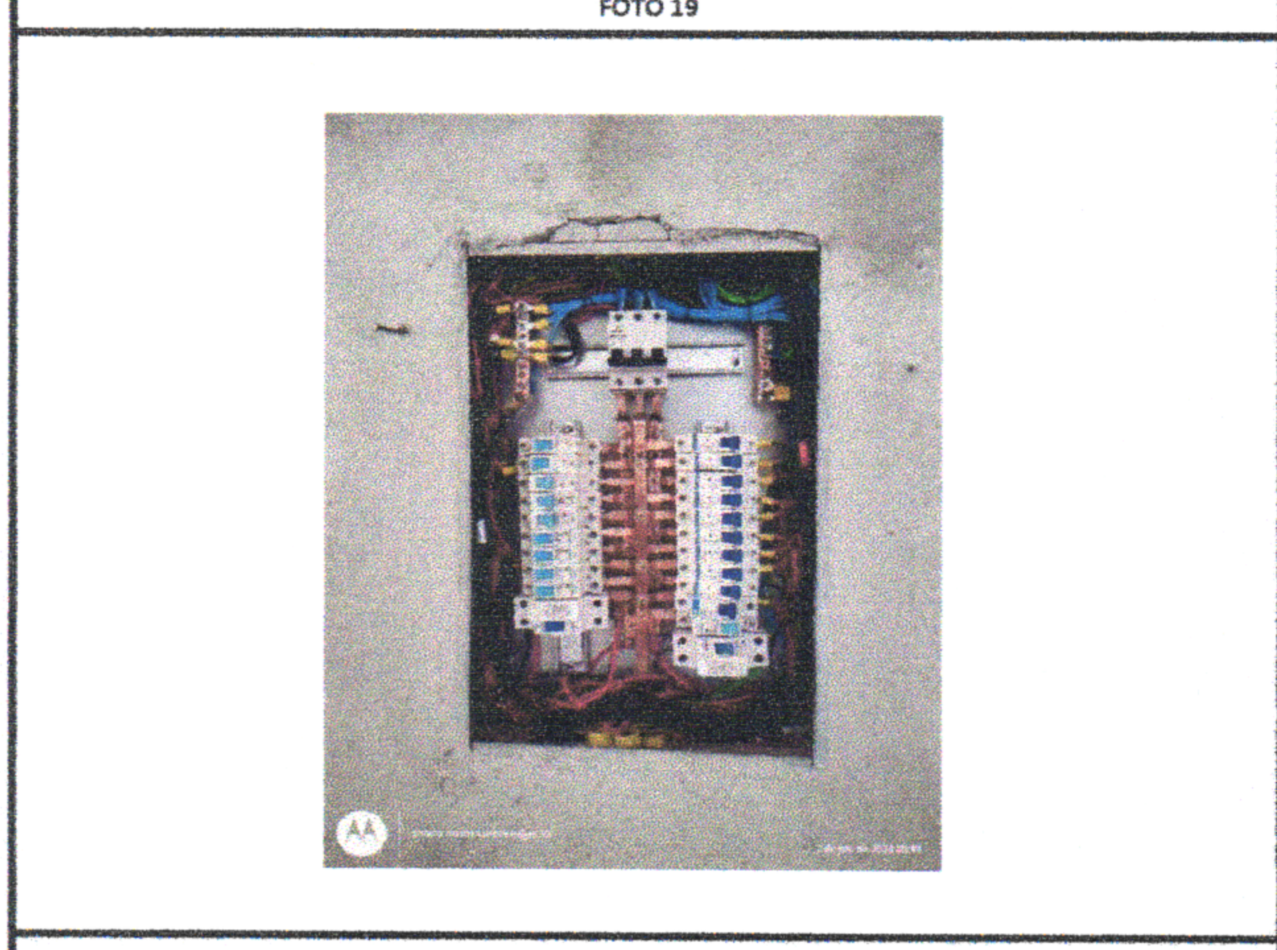
1.9.29 - DISJUNTOR MONOPOLAR TIPO DIN, CORRENTE NOMINAL DE 25A - FORNECIMENTO E INSTALAÇÃO. AF_10/2020
