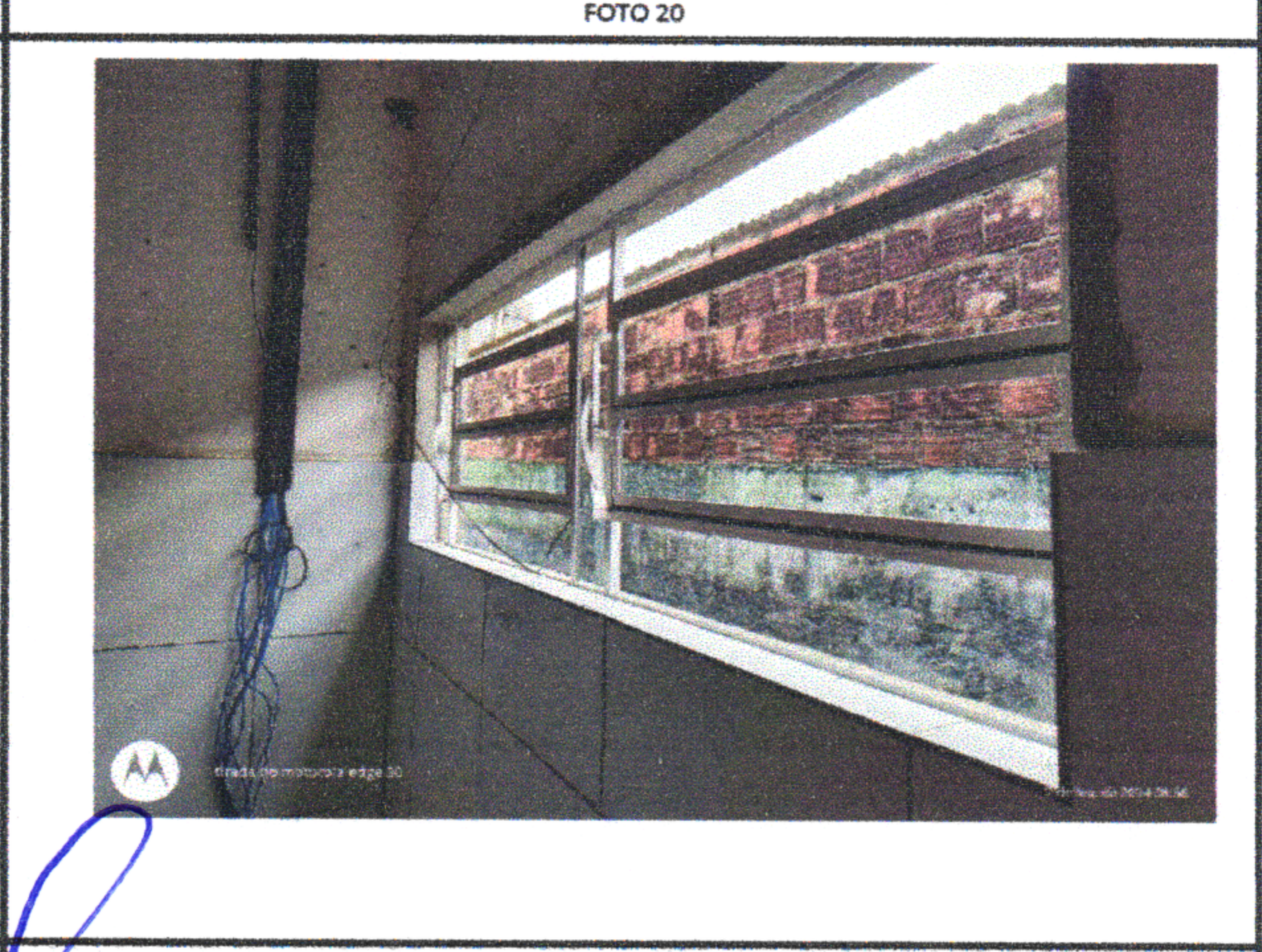
1.10.10 - PONTO PARA CABEAMENTO ESTRUTURADO EMBUTIDO, COM ELETRODUTO DE PVC RIGIDO Ø 3/4" C/CABO UTP 4 PARES CAT. 6
