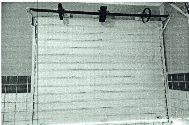
PORTA DE ENROLAR DA COZINHA
