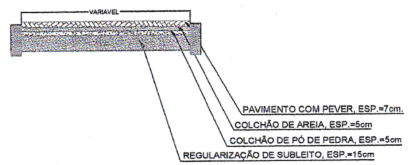
SEÇÃO TÍPICA DA 2ª TRAVESSA ALDERITA EVANGELISTA
