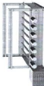
Itagrill Dupla Linear 7 Espetos * Espetos Espadas Altura: 28,5 cm Profundidade: 65,0 cm Frente: 48,5 cm Frente com Motor: 58,5 cm Código: 9326
