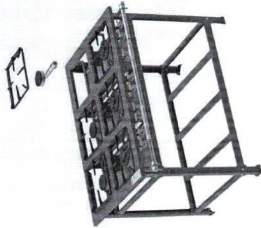
Fogão 6 Bocas 3 Q. Duplos e 3 Q. Simples Altura: 80,0 cm Profundidade: 86,5 cm Frente: 150,0 cm Código: 6028
