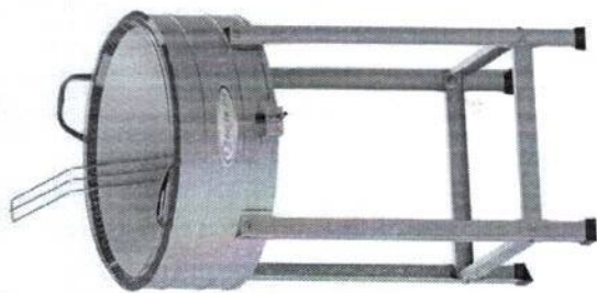
Fritador Médio Inox Gás Cesto Vendido Separado Altura: 84,5 cm Diâmetro: 45,0 cm Código: 10003-1 Código Cesto: 137
