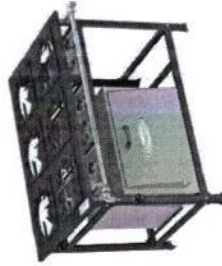
Fogão 6 Bocas 6 Q. Simples AP Altura: 80,0 cm Profundidade: 88,5 cm Frente: 117,0 cm Código: 6011 / 9017
