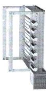
Itagrill Dupla Linear 7 Espetos * Espetos Mistos Altura: 28,5 cm Profundidade: 65,0 cm Frente: 48,5 cm Frente com Motor: 58,5 cm Código: 9323
