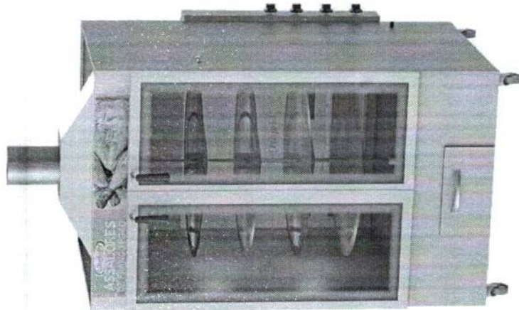
FG40 Altura Externa: 190,0 cm Frente Externa: 99,5 cm Profundidade Externa: 112,0 cm Altura Interna: 110,0 cm Frente Interna: 83,0 cm Profundidade Interna: 89,0 cm Código: 80002
