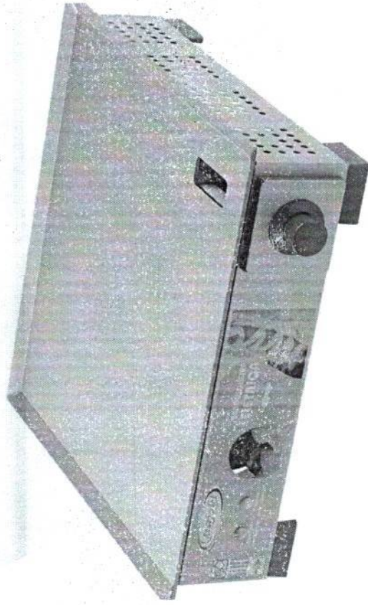
Sanduicheira 430x430 Altura: 12,0 cm Profundidade: 46,0 cm Frente: 43,0 cm Código: 11053
