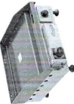
Chapa Profissional 450x470 1 Queimador Altura: 22,0 cm Profundidade: 49,0 cm Frente: 45,0 cm Código: 11011
