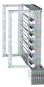
Itagrill Dupla Linear 7 Espetos * Espetos Mistos Altura: 28,5 cm Profundidade: 65,0 cm Frente: 48,5 cm Frente com Motor: 58,5 cm Código: 9323
