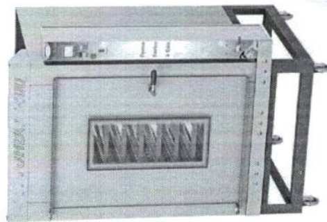
Forno Digital 1400 Capacidade 10 Esteiras Altura: 173,0 cm Profundidade: 128,5 cm Frente: 104,0 cm Código: 55006
