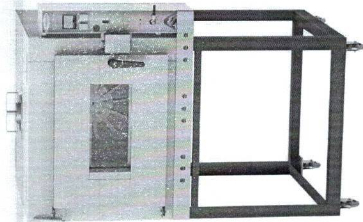
Forno Digital 900 Light Capacidade 5 Esteiras Altura: 173,0 cm Profundidade: 128,5 cm Frente: 106,0 cm Código: 55007
