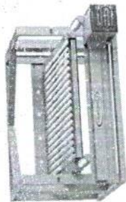
Elevante 5 Espetos com Motor Altura: 43,5 cm Profundidade: 64,5 cm Frente: 75,0 cm Código: 9390
