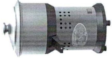
Extrator Plus Inox Caçamba Alumínio Bica Plástica 1/4 Cv Altura: 33,5 cm Diâmetro: 19,0 cm Código: 70004-4
