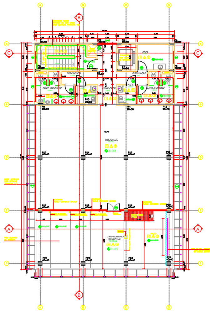
4º PAVIMENTO esc:1:150
